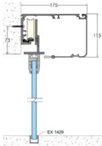
Guía empotrada
